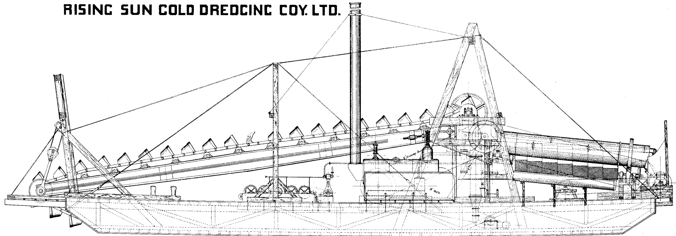
ELEVATION
